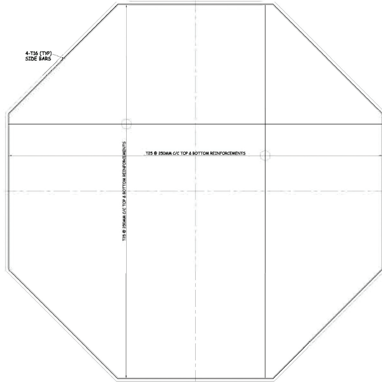
SECTION - DD
